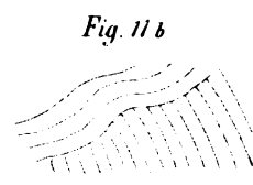
Fig. 11. Vierte Hypothese über die Entstehung des Mettenbergs.
